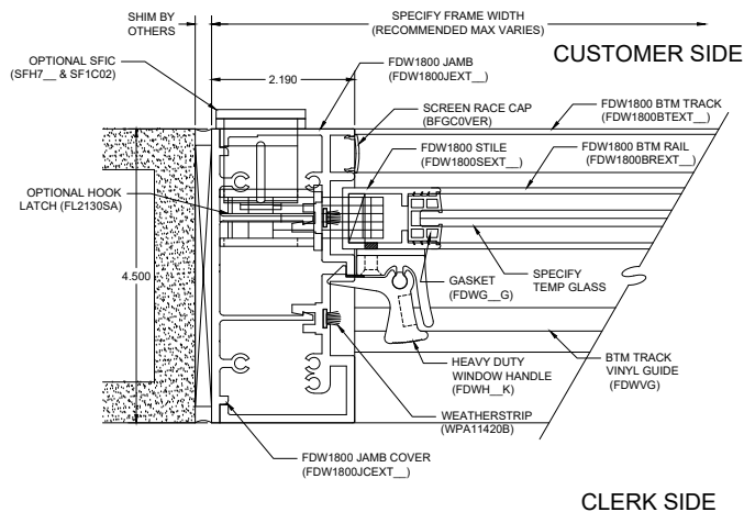
C4 JAMB & WALL DETAIL
