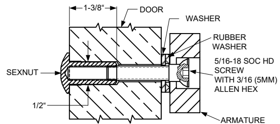
FIG. 2B SOLID DOOR
